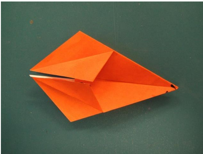
⑰上部を一枚めくり平らな部分が出るようにする。⑱綴じている側の頂点を中央部分に向けて折る
